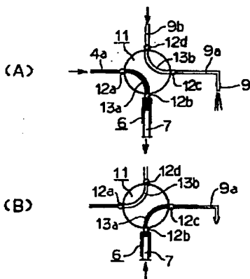
本発明の第二の実施の形態を示す流路図
